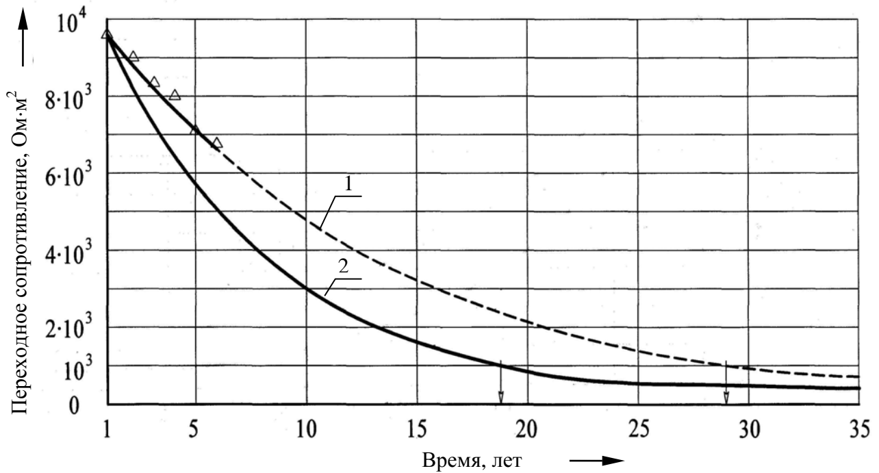
Рис. 12. Изменение переходного сопротивления R_{п} образцов изолированных труб:
