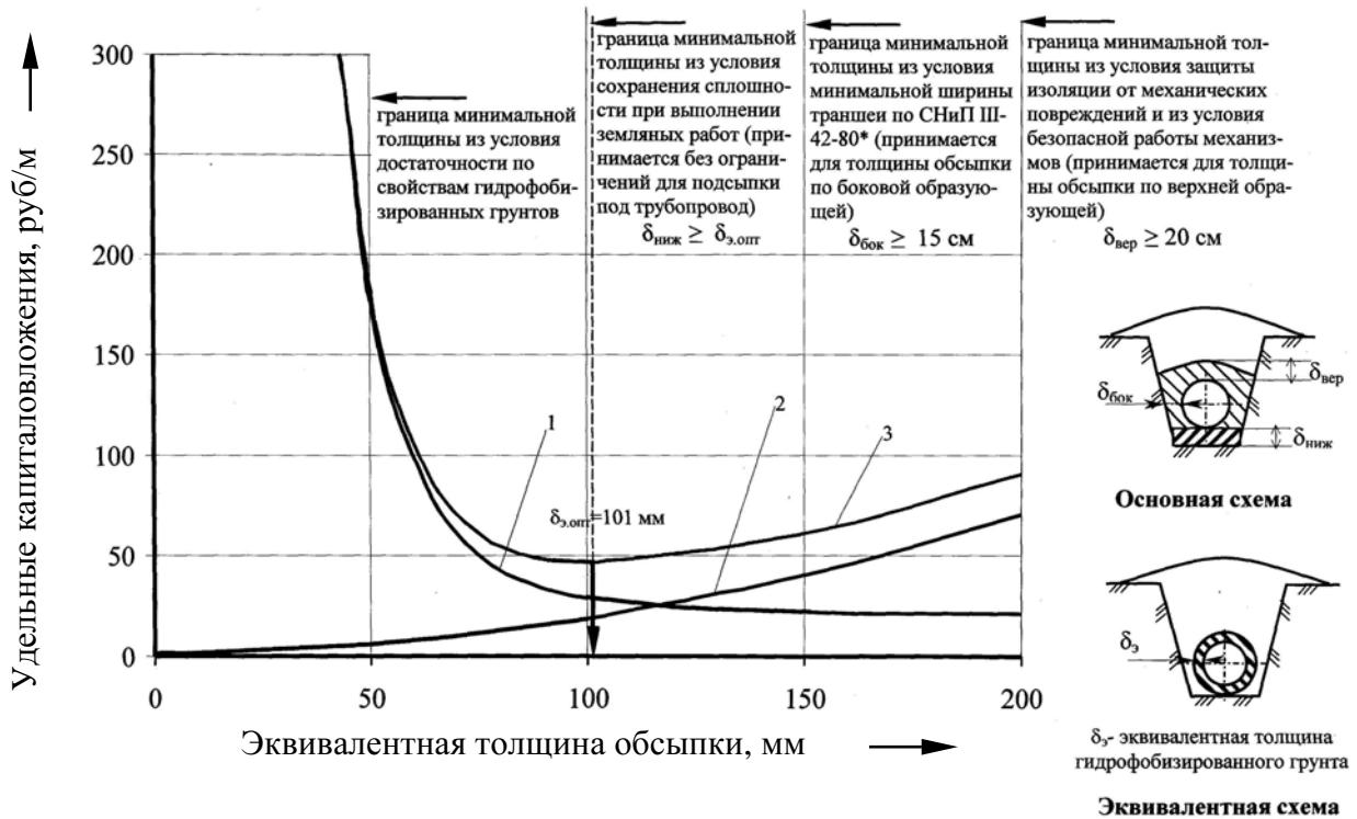
Рис. 10. Определение оптимальной толщины обсыпки из ГФГ по целевой функции: 1 – стоимость ремонта изоляции (в ценах 1984 г.); 2 – стоимость обсыпки ГФГ с эквивалентной толщиной \delta_3 (в ценах 1984 г.); 3 – целевая функция для нахождения оптимальной толщины обсыпки
