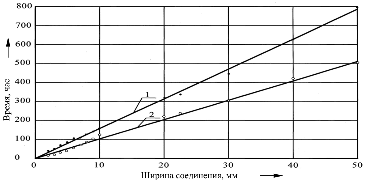
Рис. 15. Зависимость водопроницаемости в нахлесте для полимерной изоляционной ленты «Полилен» при 90 °С:
