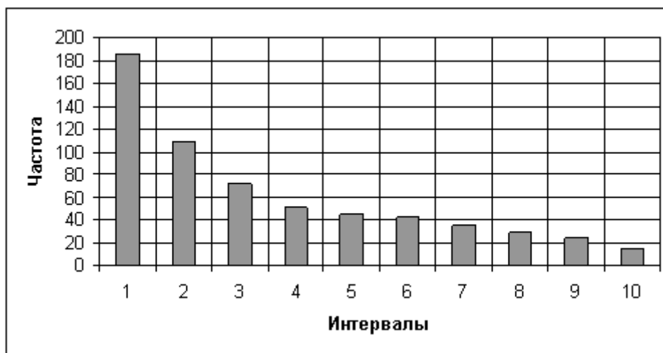
Рисунок 2. Гистограмма распределения колебаний показателей эффективной вязкости нефти
