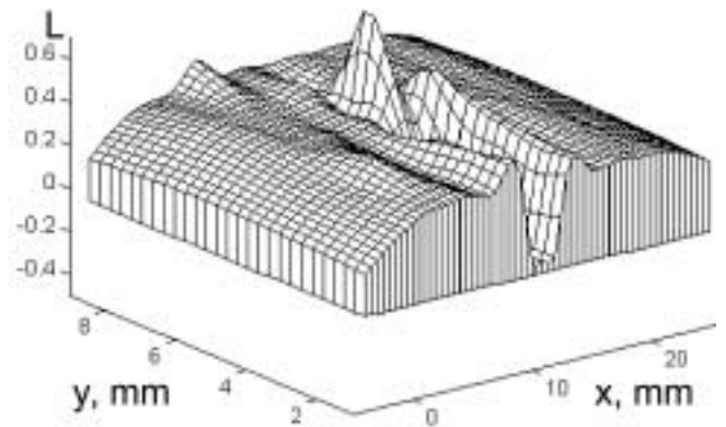
Рис. 7. Рельеф параметра поврежденности L в области пластических деформаций
