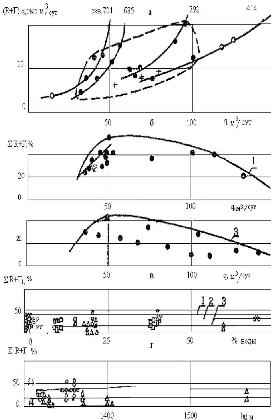
а - эффективная область применения диспергаторов для 4-х штуцеров диаметром 20 мм на глубины 1350 м; б, в и г - влияние дебита, обводненности и глубины установки диспергатора на снижение расхода газа, количество: 1-4; 2-3; 3-2 - диаметр штуцеров 20 мм
