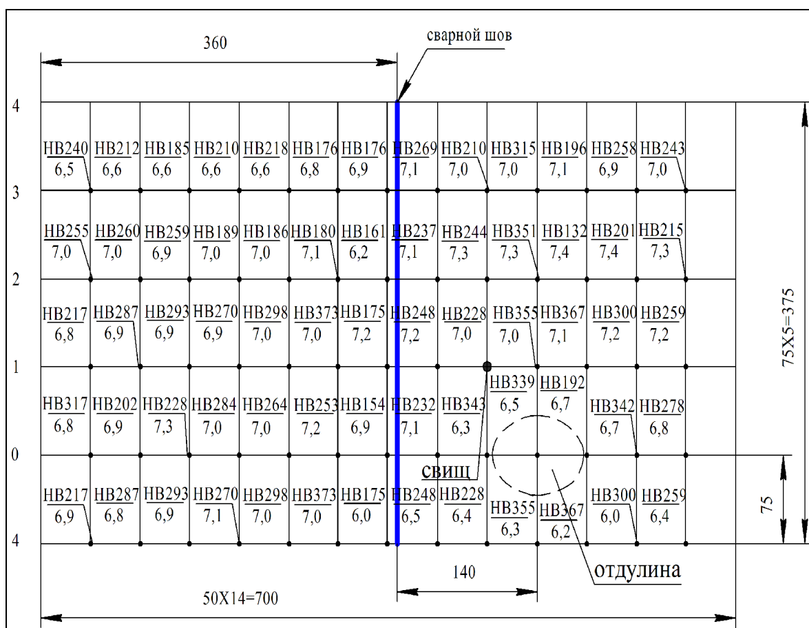
Рисунок 3. Развертка фрагмента трубы с замераами твердости и толщин стенки по зонам 0-4
