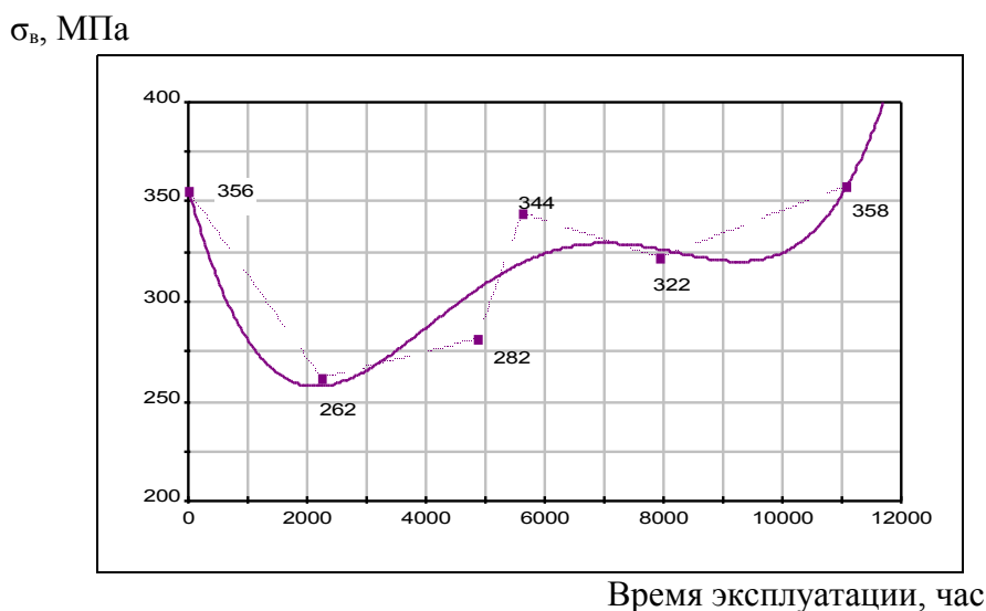
Рисунок 2. Изменение предела прочности стали 20X23H18 в процессе эксплуатации в пиролизной печи
