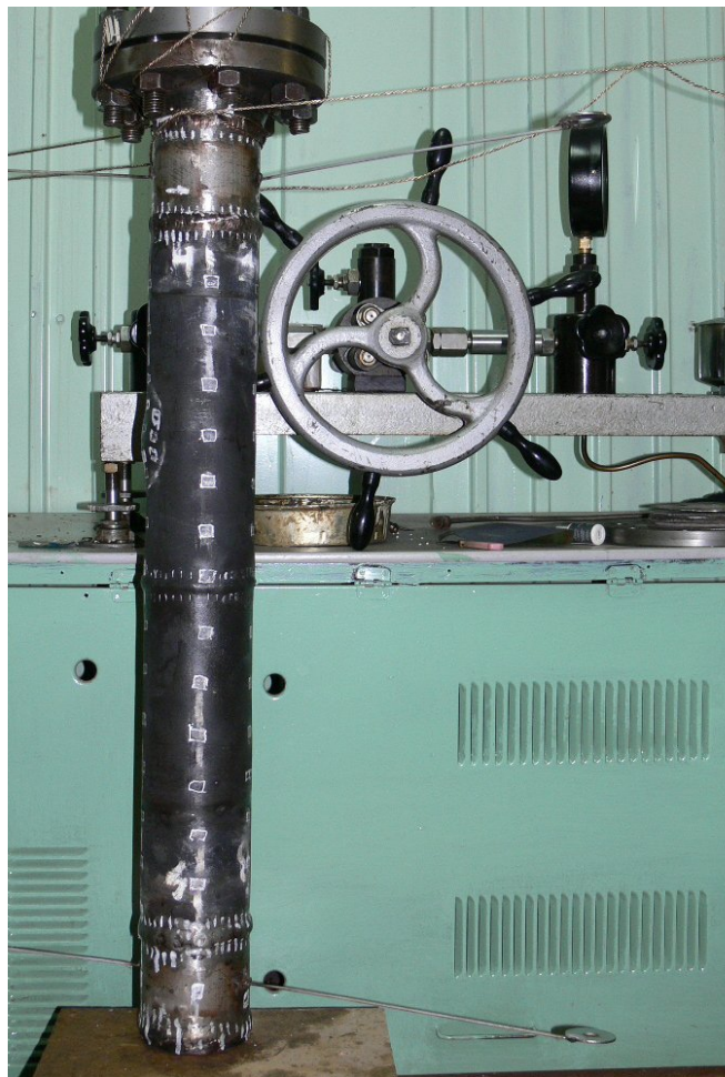
Рисунок 6. Общий вид испытательной установки с сосудом
