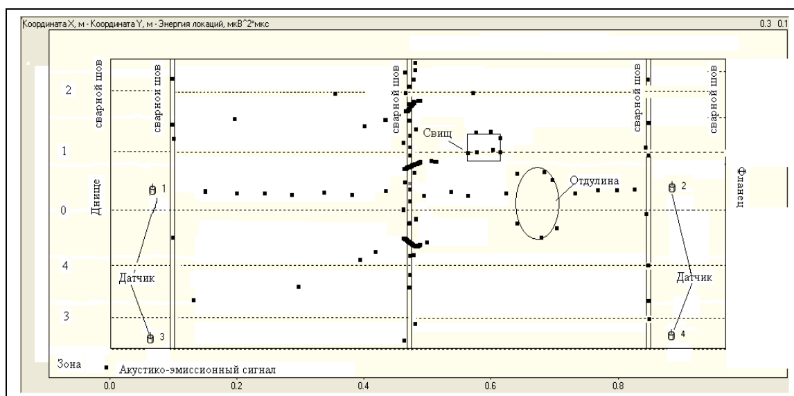
Рисунок 9. Образование свища при достижения давления 33 МПа
