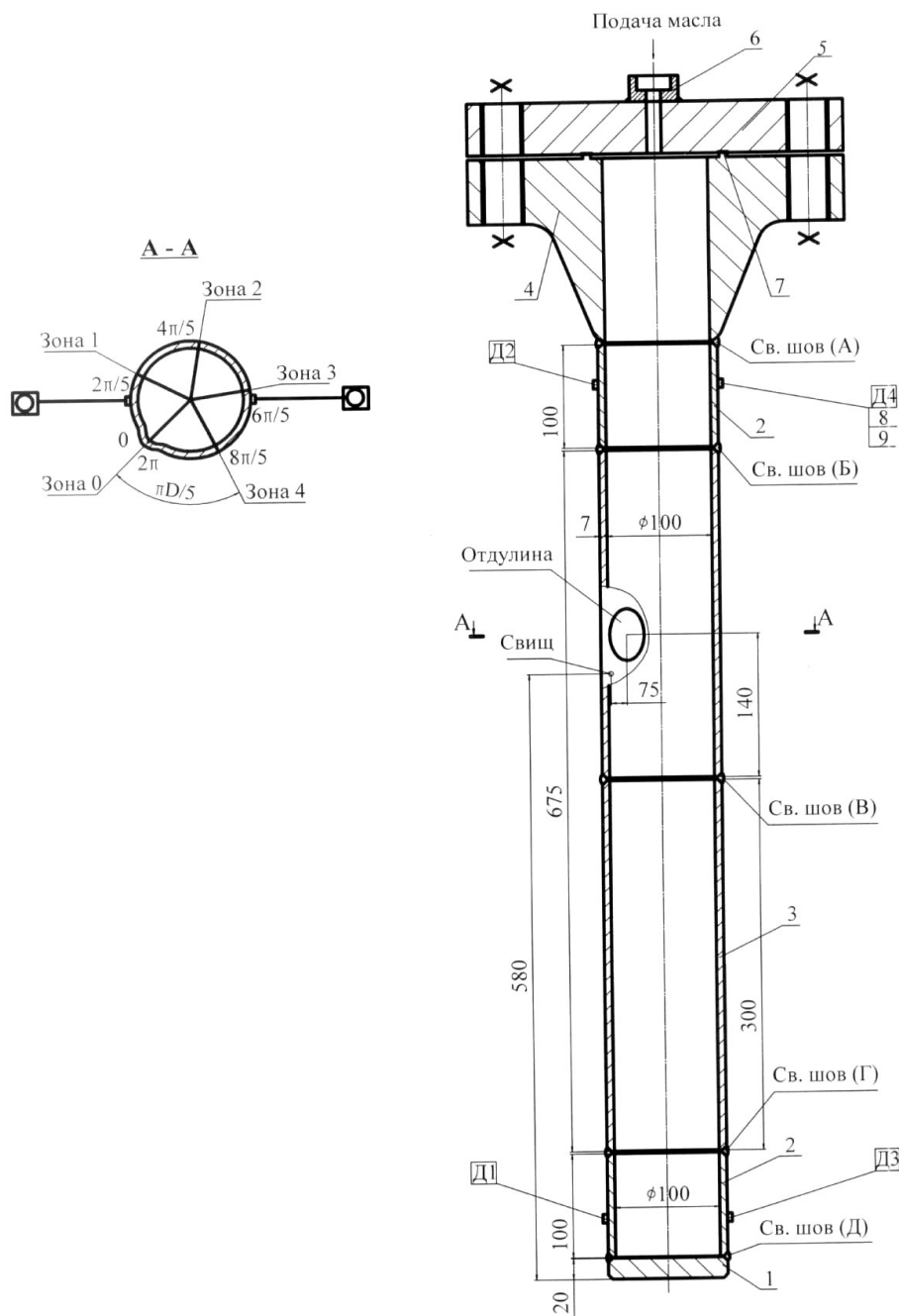
Рисунок 5. Сосуд цилиндрический для испытания внутренним давлением:
